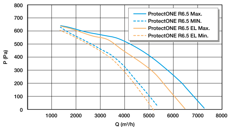
Caractéristiques aérauliques ProtectONE® R 6.5 - 1V
